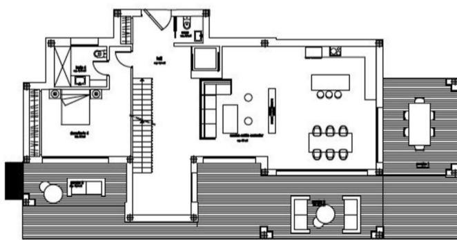
planta baja
